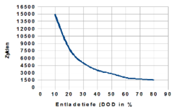
Lebensdauer@ Entladetiefe
